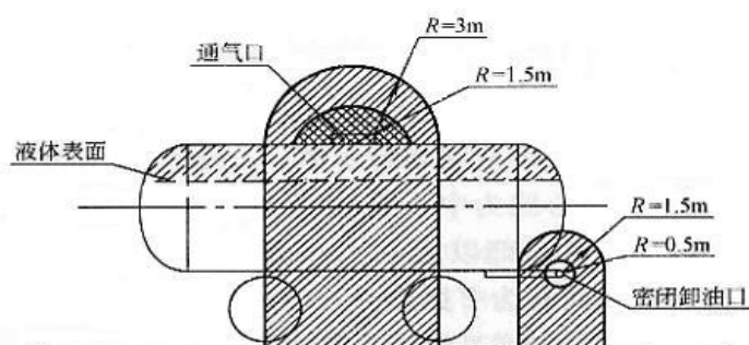
附图 2 油罐车和密闭卸油口爆炸危险区域划分
